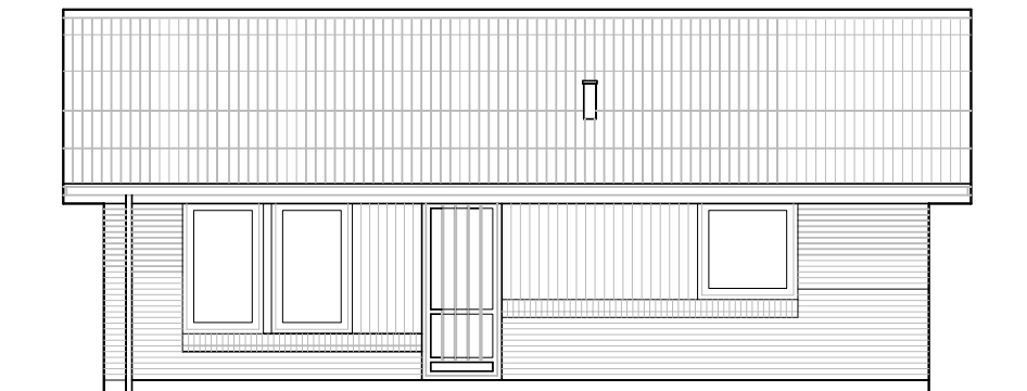
Facade fra havesiden – Type 77 – Retvendt.
