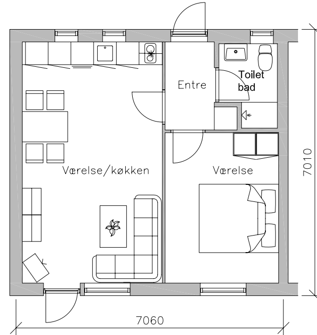
Plantegning - 2 værelse 50m 2 Ret til ændringer forbeholdes.
