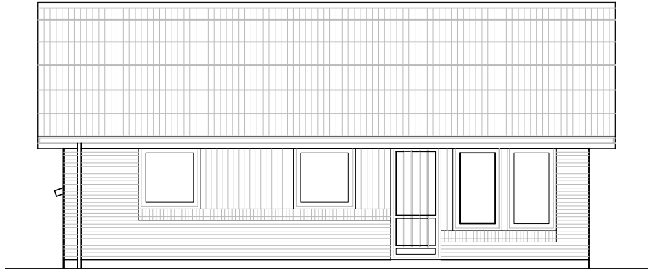
Facade fra havesiden – Type 99 – Spejlvendt.
