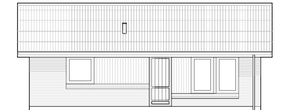
Facade fra havesiden – Type 77 – Spejlvendt.
