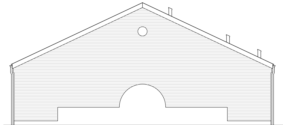
Gavl - Type 95+1 - Retvendt
