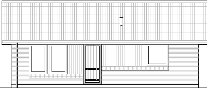
Facade fra havesiden – Type 77 – Retvendt.
